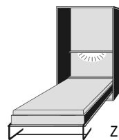
Schrankbett(ohne Matratze) mit LED-Beleuchtung unter Ablageboden mit fest eingebautem Lattenrost, Härtegradeinstellung im Mittelteil, Matratzenhöhe maximal 20cm
